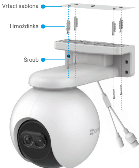
Obr. 1 Montáž na strop
